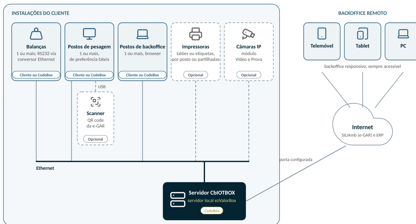
Instalação modelo de um posto de pesagem
